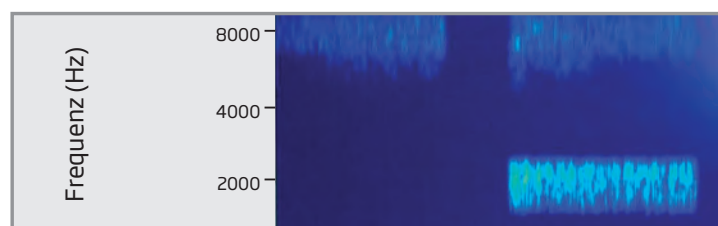
Abb. 4 Links bzw. rechts ist das Spektrum für den Laut „s“ ohne bzw. mit Speech Rescue dargestellt.
