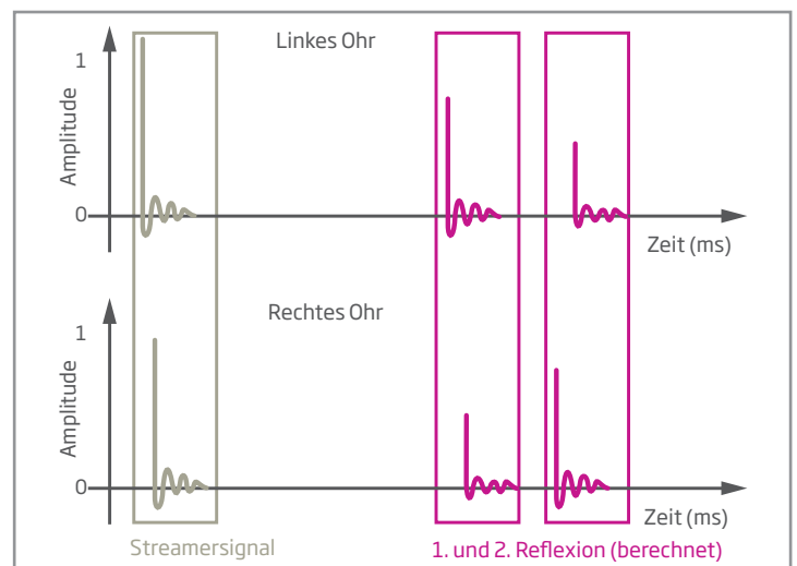
Abb. 4: Der Schall vom Streamer wird bei Musik-Panorama ergänzt durch rechnerisch ermittelte Reflexionssignale. Diese werden durch binaurale Signalverarbeitung links und rechts unterschiedlich berechnet.
